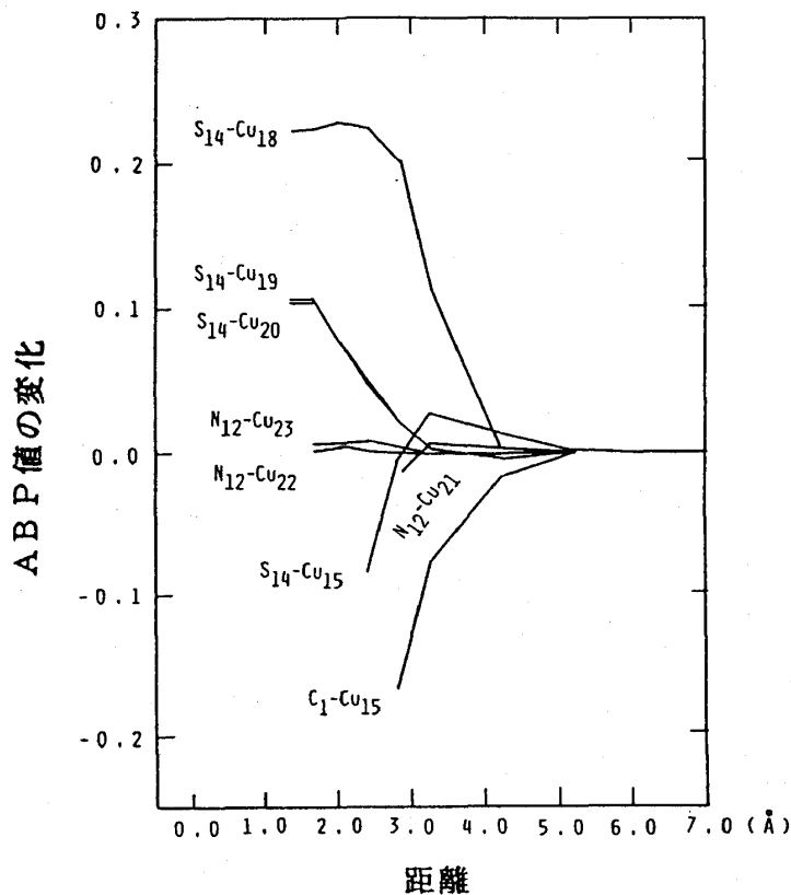
図2 MBT - の S_{14} と N_{12} とCu(100) 13 第1層のCuとのAOBP値
