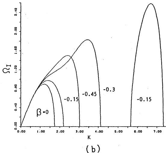
図 1. (a) \beta に対する不安定領域 K_c と (b) K に対する増幅係数 \Omega_I .
