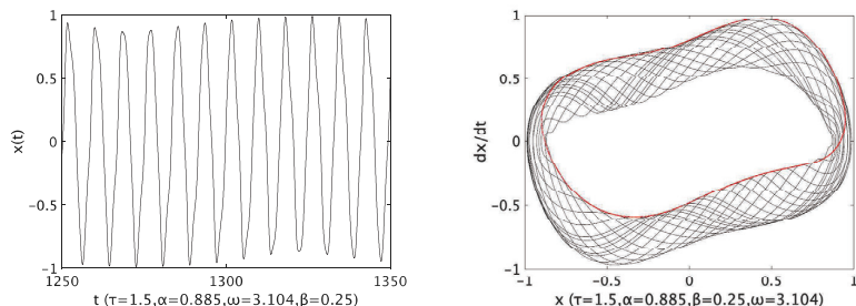
図 4. オイラー法によって近似計算した概周期解 ( \tau = 1.5, \alpha = 0.885, \beta = 0.25, \omega = 3.104 )
