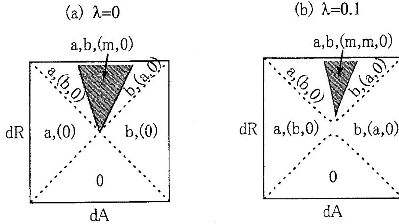
図 8: 平衡解の存在領域. 点線は中立曲線を表す. 0, a, b, m はそれぞれ自明解, a モード, b モード, 混合モードを表す. かつこのないものは安定な解, かつこの内ものは不安定な解である. \mu_2 = 2, \mu_3 = 3 .
