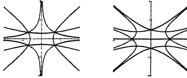
図 1: Stokes 曲線と反 Stokes 曲線。左は P(x, E) = x^4 + 1 ( E = -1 )、右は P(x, E) = x^4 - 1 ( E = 1 ) のもの。
