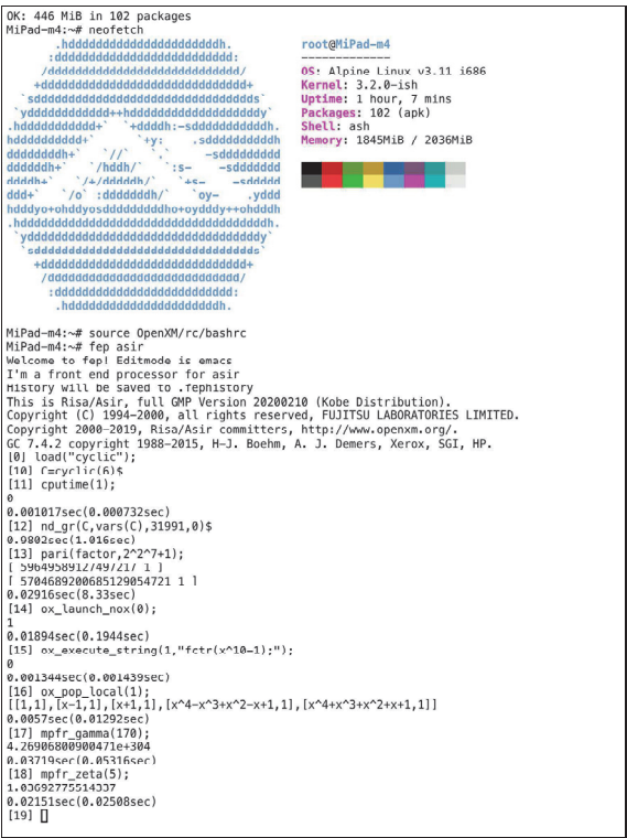
図 2: iSH Shell で動作する Risa/Asir
