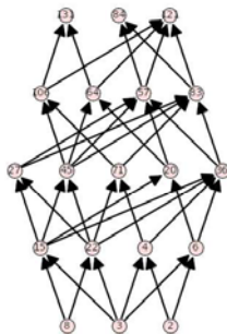
図 5: \mathcal{J}_6^{\text{HTS}} のハッセ図
