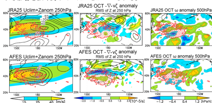
図 3: 上段が観測、下段がモデルにおける 10 月の図。(左)250hPa での背景の西風風速(色)と高度偏差(黒線)、(中)250hPa での移動性擾乱に伴う高度場の RMS 偏差(黒線)と渦度フラックス収束による渦度変化傾向偏差(色)、(右) 500hPa の鉛直流偏差。
