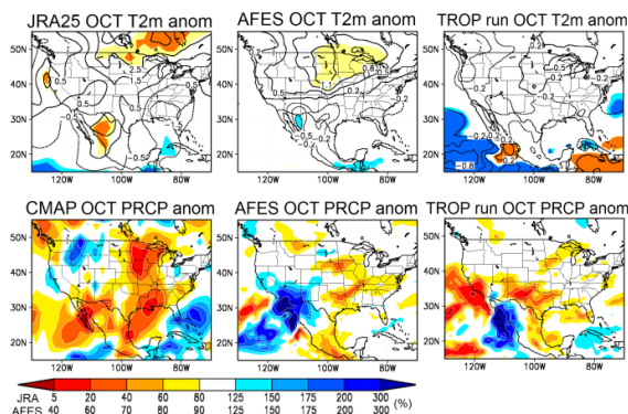
図 6: 10 月における海面水温偏差(上段)と 250hPa 高度偏差(下段)。左は中緯度実験、右は熱帯域実験の結果を示す。色は 95%有意な偏差を示す。
