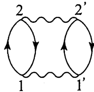
図 11: 2次摂動の Feynman 図形の一つ
