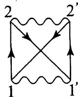
図 12: 2 次摂動における別の Feynman 図形
