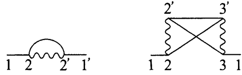
図 17: 松原グリーン関数に寄与する Feynman 図形の例
