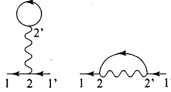
図 4: \check{G} に寄与する 1 次の Feynman 図形
