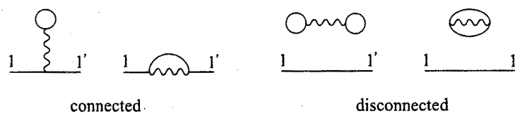
図 16: 松原グリーン関数に対する 1 次の Feynman 図形
