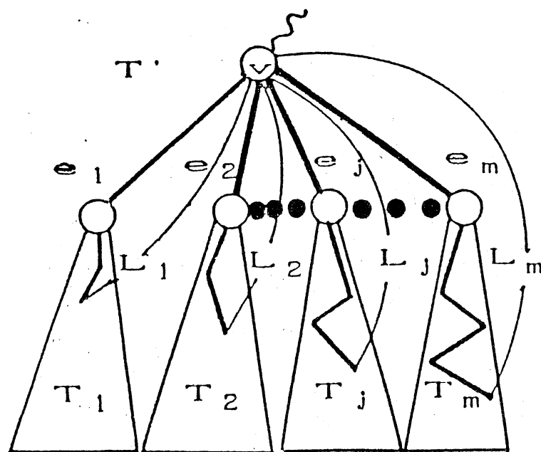
図3. k 鎖の木への節点パッキング.
