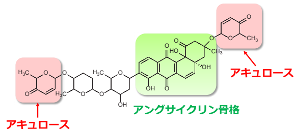
図. 2 サプロルマイシン E の構造
