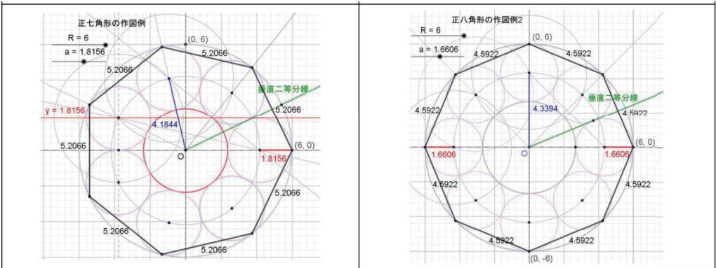
図 5: 左側 正七角形の作図例 右側 正八角形の作図例
