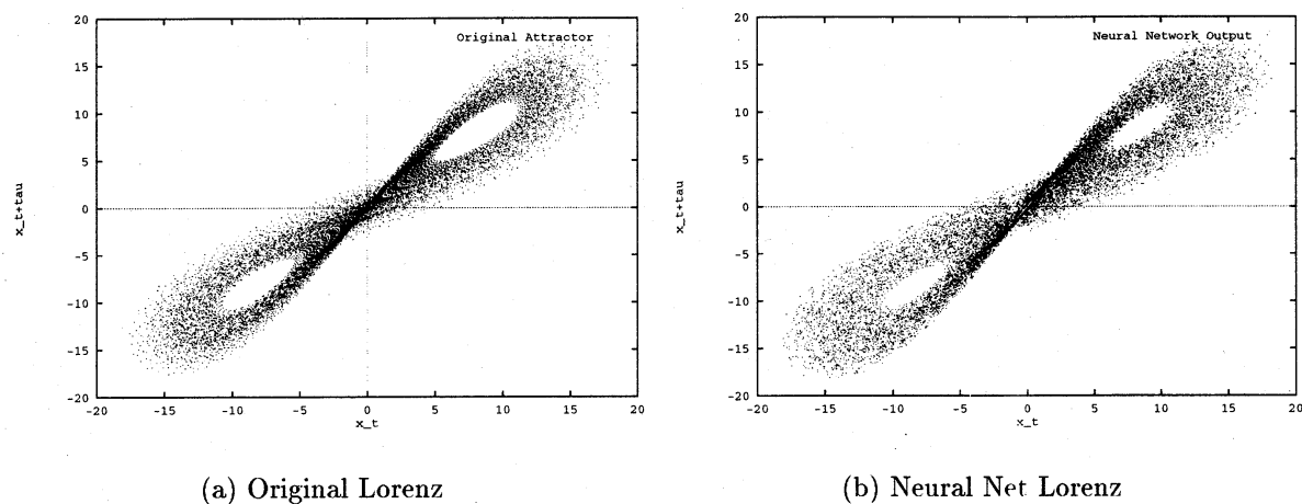
図 4.6 (x_t, x_{t+\tau}) 空間のアトラクタ比較
