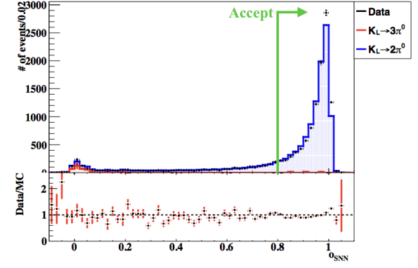
(d) o_{\text{SNN}}
