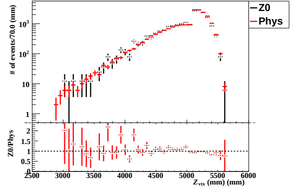
(f) Z_{\text{vtx}}
