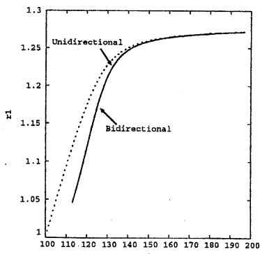
図6: r_1^* の比較
