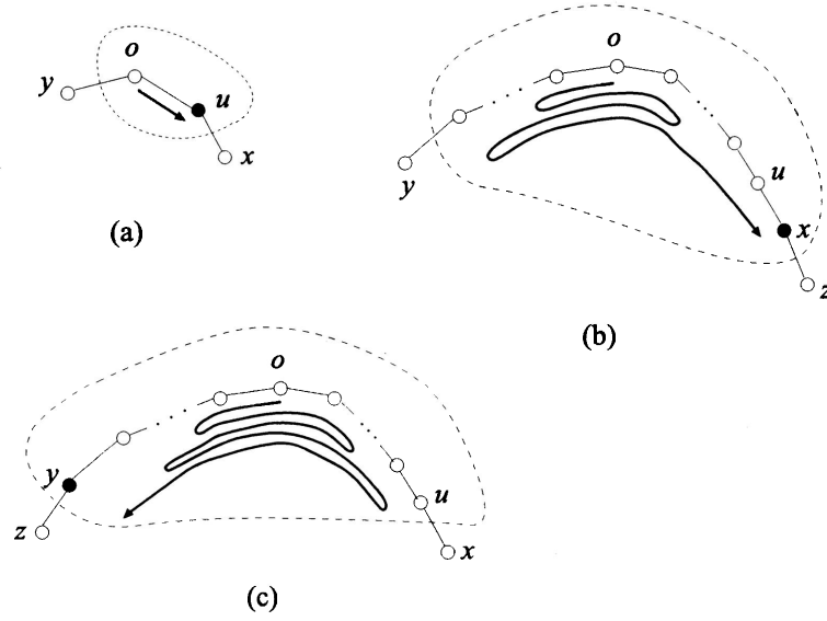
図 4 補題 1 の証明
