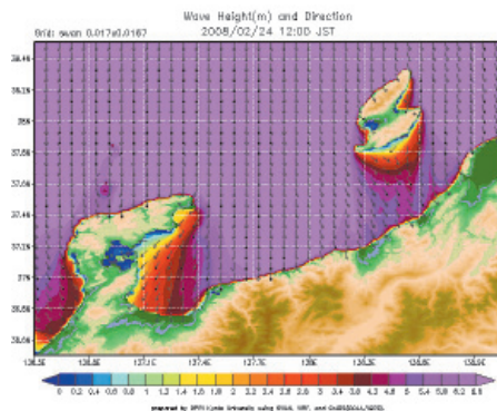
図 1 SWAN による冬季風浪のシミュレーション
