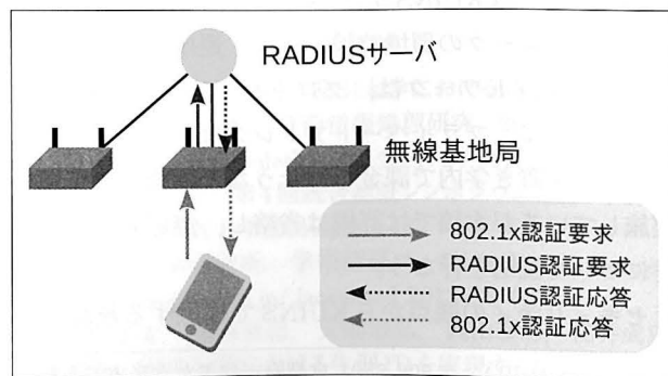
図3. 自機関でeduroamを利用する際の認証
