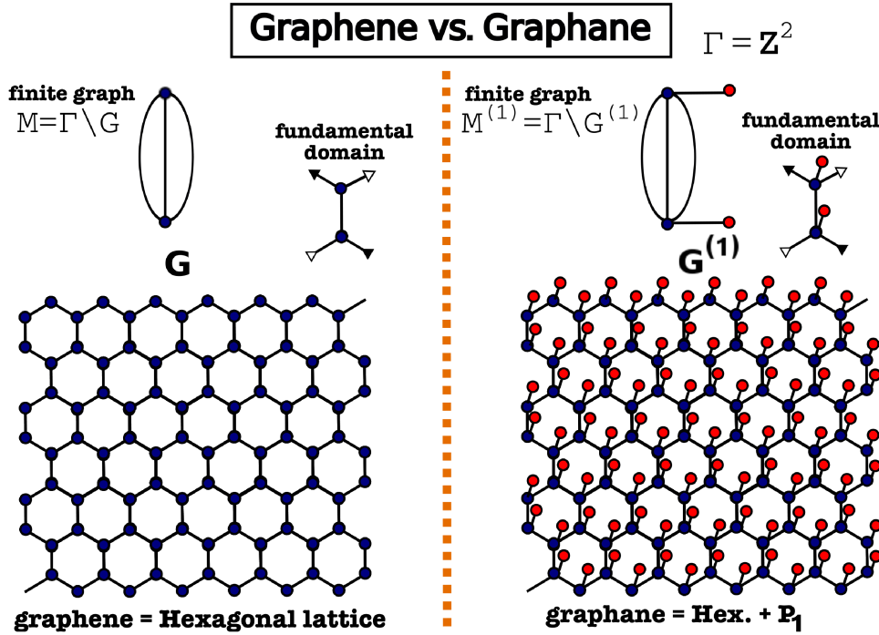
Figure 2. グラフとしての graphene G と graphane G^{(1)} .
