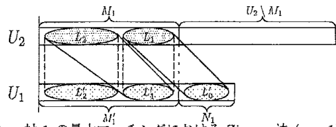
図 2: s 対 1 の最大マッチングにおける Zigzag 法 ( s=1 )
