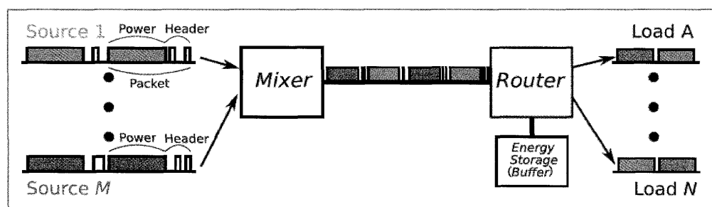
図-6 電力パケットとルータ
