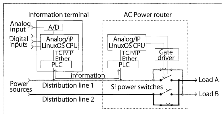
図-8 ac ルータの構成
