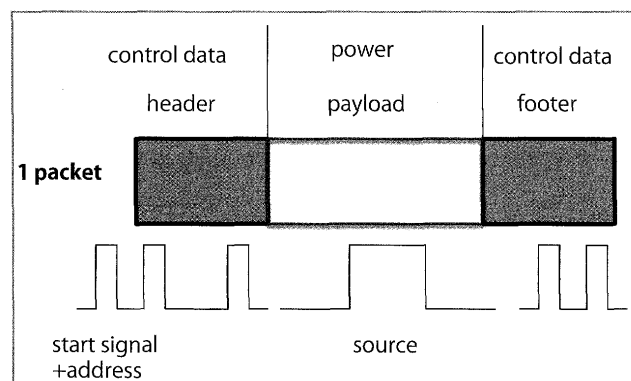
図-7 電力パケットの構成
