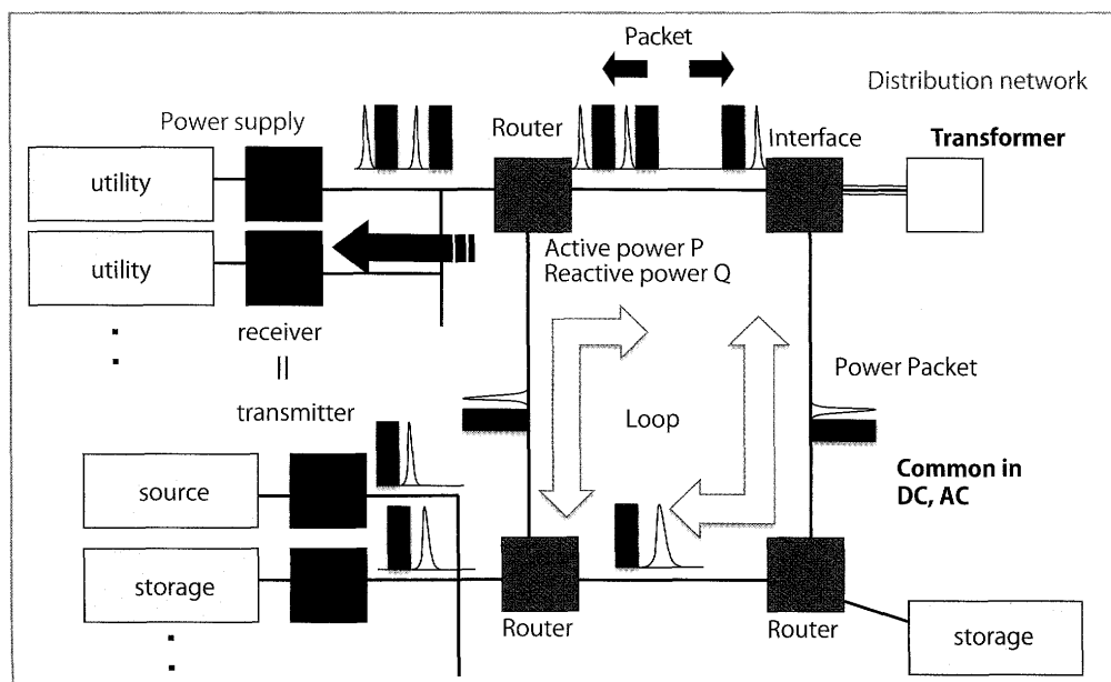
図-5 Home Network における電力パケットの伝送
