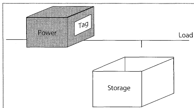
図-1 電力パケットの概念
