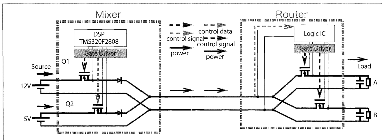
図-9 dc ルータの構成
