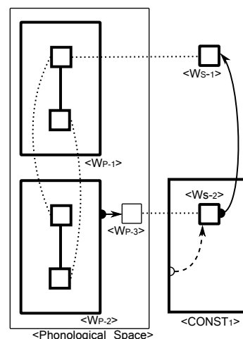
図 4.15: かすり (APEU)
