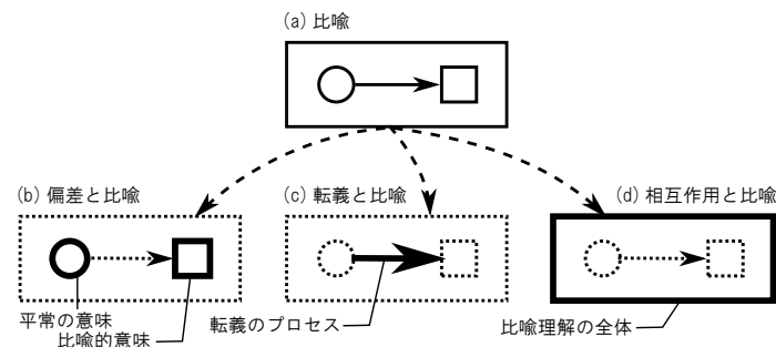
図 2.1: 比喩の諸相
