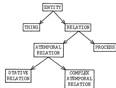
図 3.3: Langacker (1987: 249)
