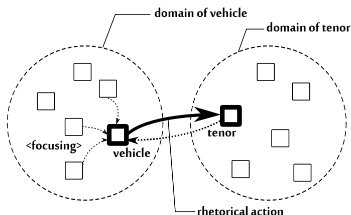
図 2.2: 修辭作用
