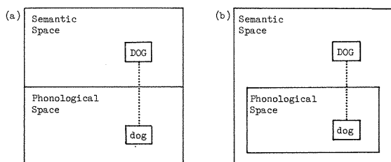
図 4.11: Langacker (1987: 80)
