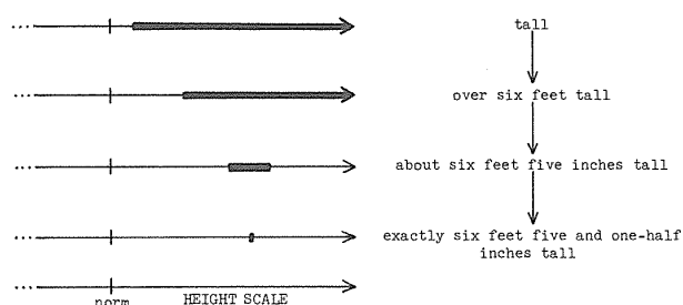
図 4.17: Langacker (1987: 133)
