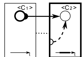
図 4.45: 格転換 (ENLAGE-antip)
