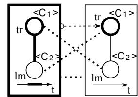
図 4.51: 代換 (HYPL)
