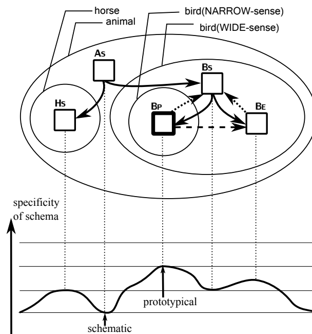
図 3.10: 地形モデル
