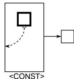
図 4.43: 黙説 ( APOSIO )
