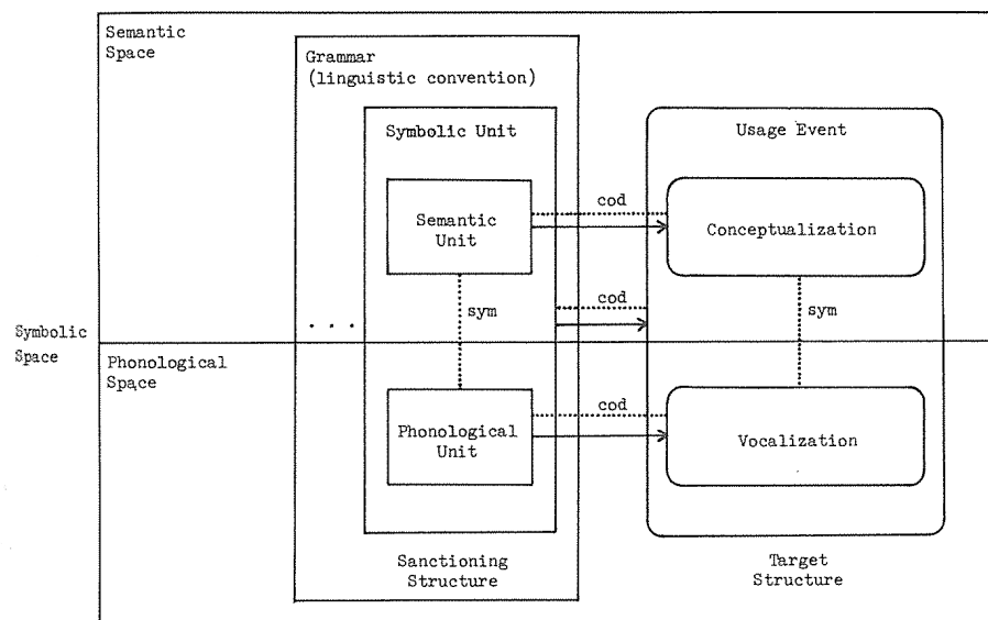
図 3.1: Langacker (1987: 77)
