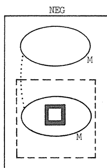
図 4.21: Langacker (1991: 134)
