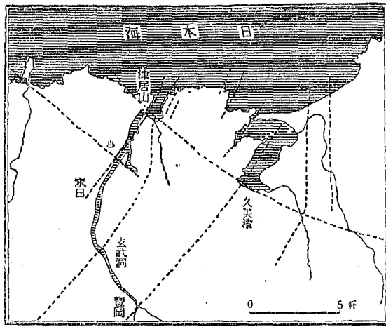
第二圖 北但馬の斷層線
