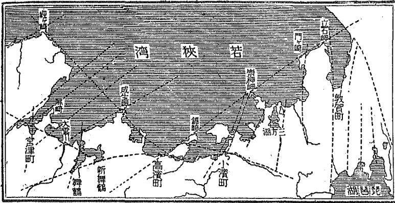
第三圖 若狹灣斷層線 0 20 40 60 米
