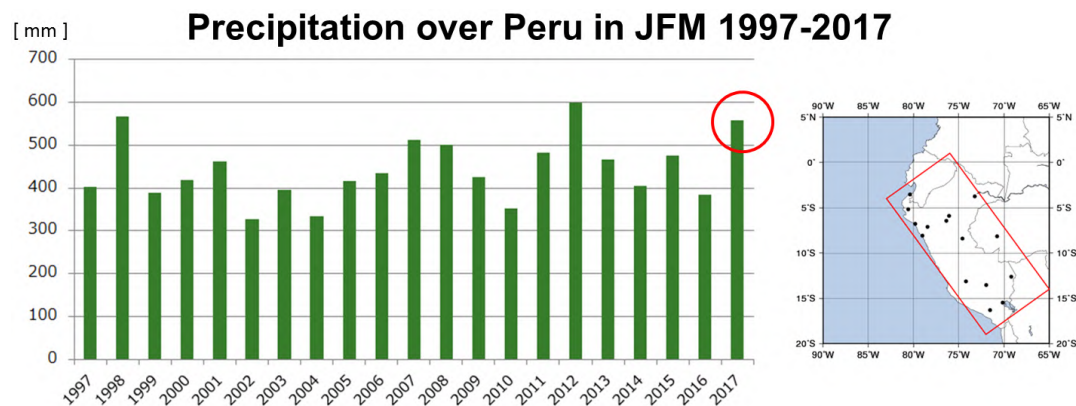
第5図 1997年～2017年の各年における1月～3月の積算降水量 (mm)。(右図赤い四角内の地点のSYNOP報を利用)
