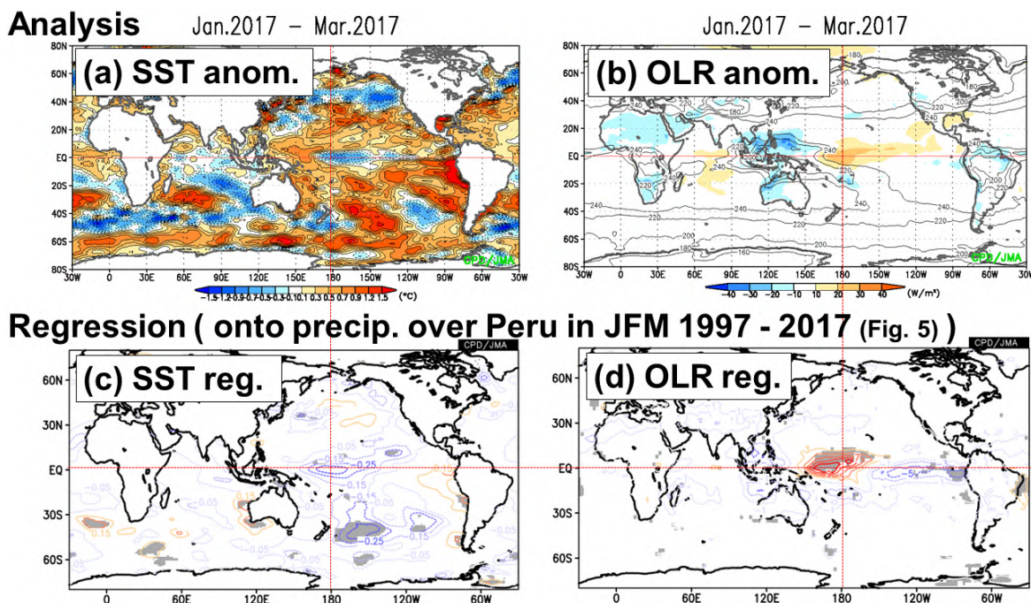
第 6 図 2017 年 1 月～3 月で平均した(a)SST 偏差 ( ^{\circ}\text{C} )、(b) OLR ( \text{W}/\text{m}^2 ) とその偏差、の解析値。1997 年～2017 年の各年におけるペルー付近の 1 月～3 月の積算降水量に対する、(c)SST 偏差、及び(d)OLR 偏差の回帰係数（コンター）。灰色の陰影は 95%信頼度水準で統計的に有意であることを示す。
