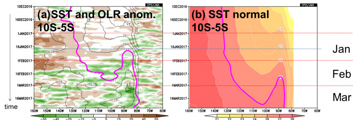
第4図 2017年1月～3月の南緯5度～10度で平均した、(a) SST (°C) (コンター) と OLR 偏差 (W/m²) (陰影)、(b) SST 平年値 (°C) (コンターと陰影) の経度時間断面図。SST27°C線を桃線で示す。
