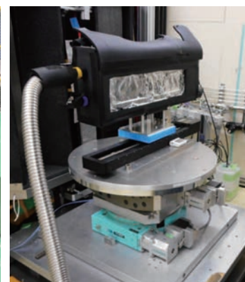
図1. 重水軽水混合調湿ガス発生装置 J-PARC 物質生命科学実験施設BL15
