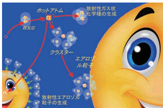
加速器室内の空气中に生成した放射性原子が最終的な生成物になるまで(イメージ)
