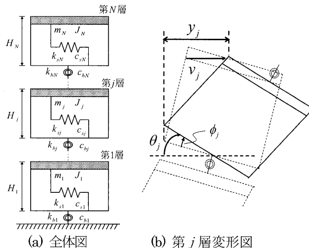
図1 N 層曲げせん断型モデル
