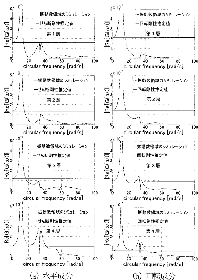
図 2 伝達関数実部の絶対値と剛性推測値
