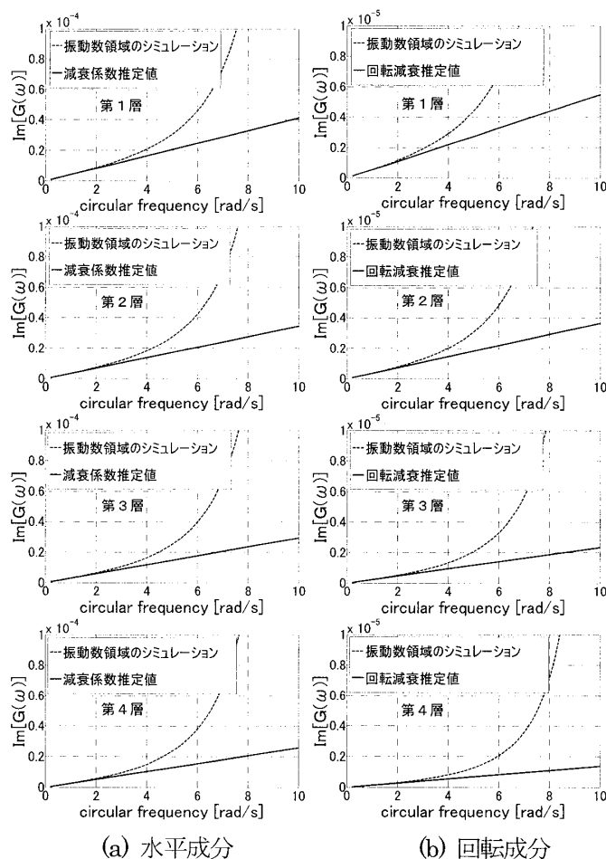
図 3 伝達関数虚部と減衰推測値
