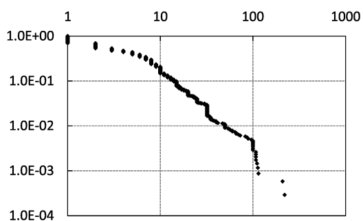
図 19: 裾確率の両対数プロット: 指値買い ( k = 9 ).
