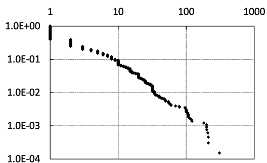
図 17: 裾確率の両対数プロット: 指値買い ( k = 8 ).
