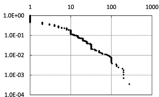
図 22: 裾確率の両対数プロット: 指値売り ( k = 10 ).
