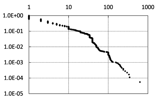
図 9: 裾確率の両対数プロット: 指値買い ( k = 4 ). 図 10: 裾確率の両対数プロット: 指値売り ( k = 4 ).
