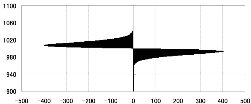
図 50: モンテカルロシミュレーションによる期待 LOB (指値注文キャンセル無し). 横軸は指値注文枚数 (正は bid, 負は ask). 縦軸は先物価格を 10 で割った値.
