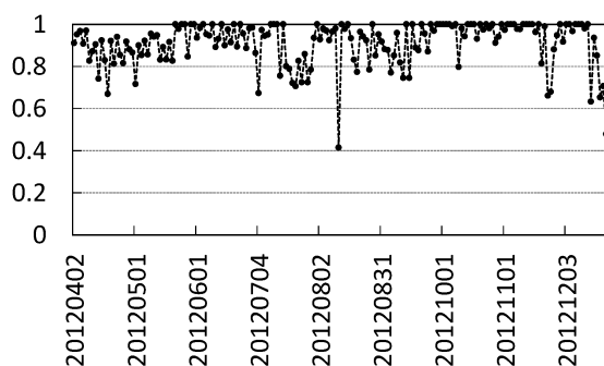
図 47: パラメーター r の時系列推移: 指値買い (図 48: パラメーター r の時系列推移: 指値売り ( k = 10 ). ( k = 10 ).
