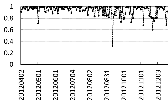
図 45: パラメーター r の時系列推移: 指値買い (図 46: パラメーター r の時系列推移: 指値売り ( k = 9 ). ( k = 9 ).
