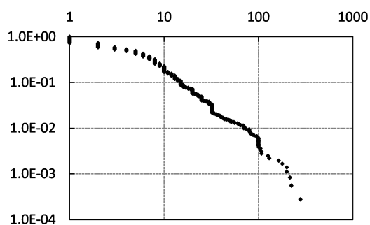
図 20: 裾確率の両対数プロット: 指値売り ( k = 9 ).
