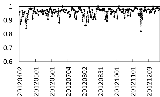
図 33: パラメーター r の時系列推移: 指値買い (図 34: パラメーター r の時系列推移: 指値売り ( k = 3 ). ( k = 3 ).
