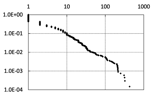
図 18: 裾確率の両対数プロット: 指値売り ( k = 8 ).
