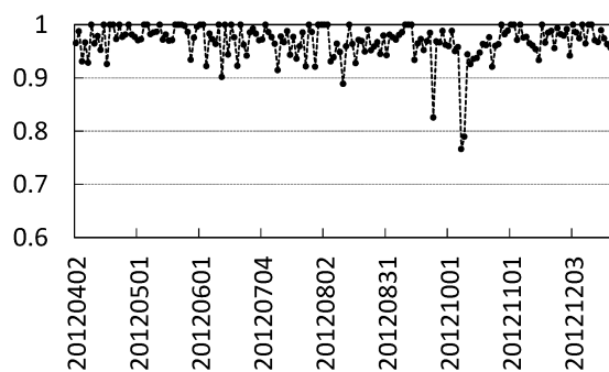
図 37: パラメーター r の時系列推移: 指値買い (図 38: パラメーター r の時系列推移: 指値売り ( k = 5 ). ( k = 5 ).
