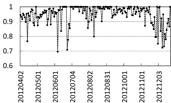
図 35: パラメーター r の時系列推移: 指値買い (図 36: パラメーター r の時系列推移: 指値売り ( k = 4 ). ( k = 4 ).
