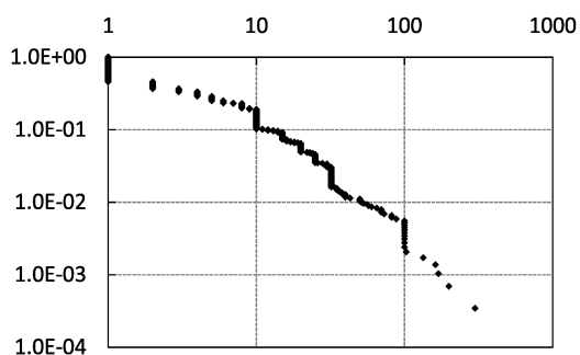
図 21: 裾確率の両対数プロット: 指値買い ( k = 10 ).
