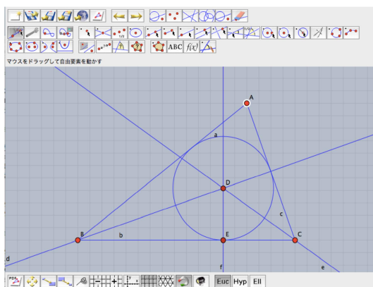
点 A を動かしても内接円は保たれる
