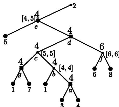
図 4: D_I(\lambda) が最大となる MPR \lambda の構築例
