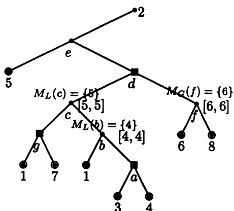
図 3: I_D(u) の構築
