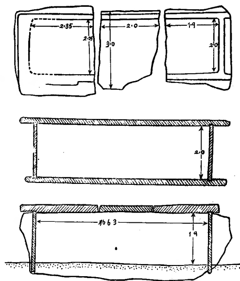
第三圖 維和村古墳石棺復原圖（梅原）
