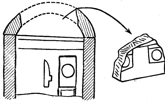
（る據に生橋午）圖棺石墳古村野吉 圖六十第
