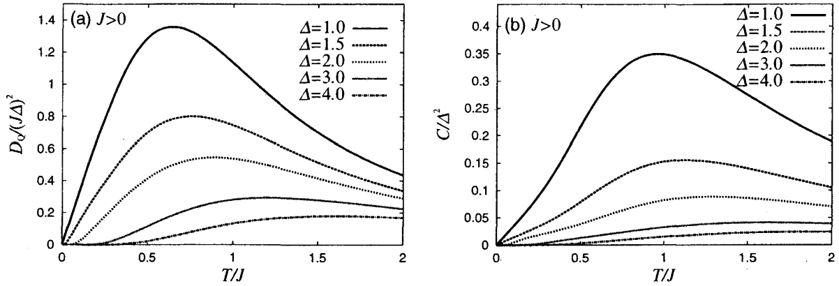
図 4.3: J > 0, \Delta > 1 における熱的 Drude 重み D_Q (a) と比熱 C (b) の温度依存性.
