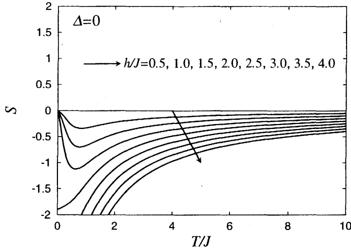
図 6.3: XY 模型 \Delta = 0 の場合の磁気的ゼーベク係数 S の温度・磁場依存性. 臨界磁場は h_c = 2J .
