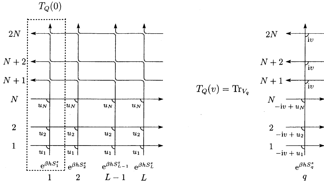
図 7.1: 左: XXZ 鎖の分配関数 Z(B.1) を図式的に表したものの。この 2 次元格子には周期的境界条件が課せられている。右: 量子転送行列 T(v) 。左図点線内で定義される量子転送行列にスペクトルパラメーター v を付加してある。
