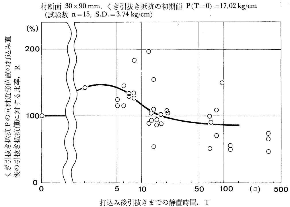
Fig. 2. 湿潤材に打ち込まれたくぎの引抜き抵抗の経時変化 (間柱材に N45 を打ち込んだ場合)
