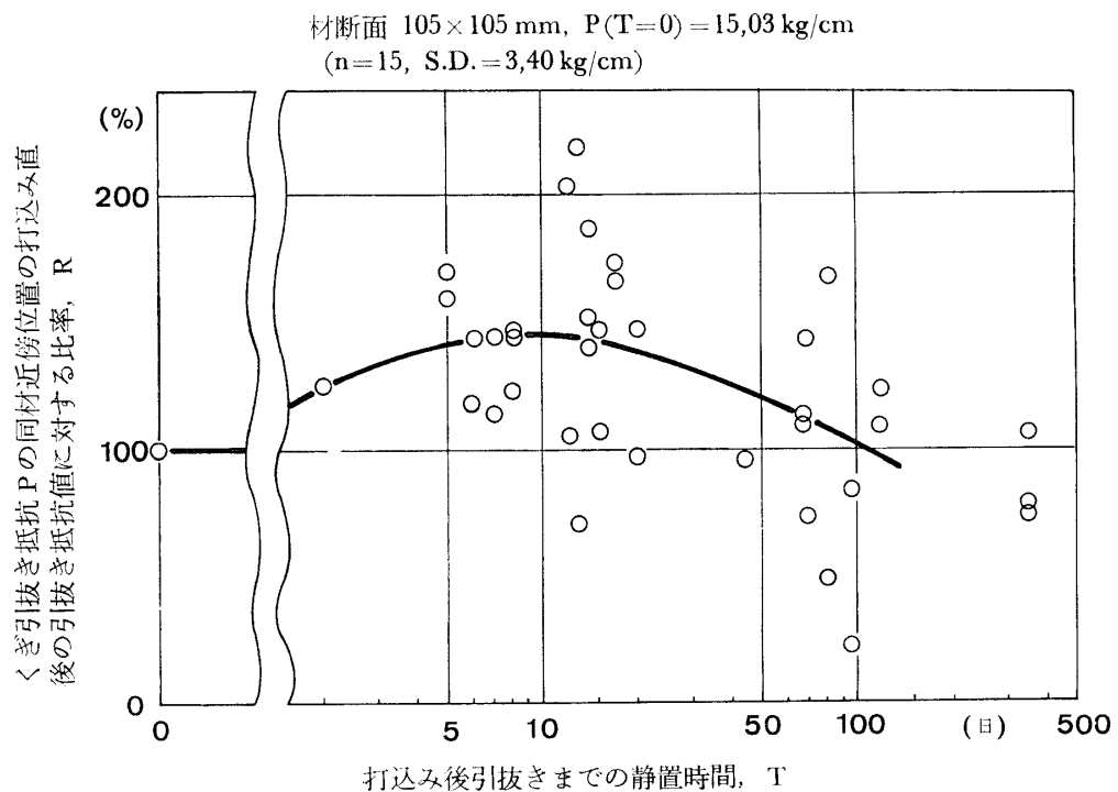
Fig. 3. 湿潤材に打ち込まれたくぎの引抜き抵抗の経時変化 (母屋角材に N45 を打ち込んだ場合)
