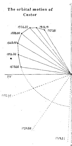
カストアの軌道運動
