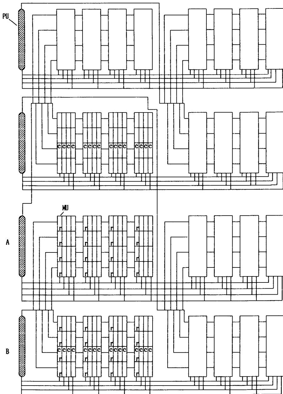
Fig. 9 (2^2, 2^3) -system
