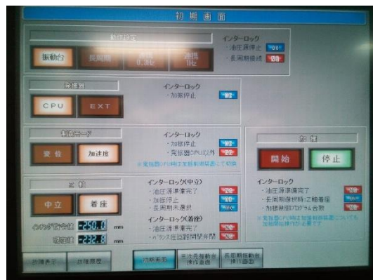
写真2 サーボ制御装置パネル
