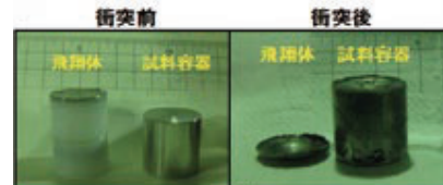
図2. 一段式火薬銃と衝突前後の飛翔体・試料容器
