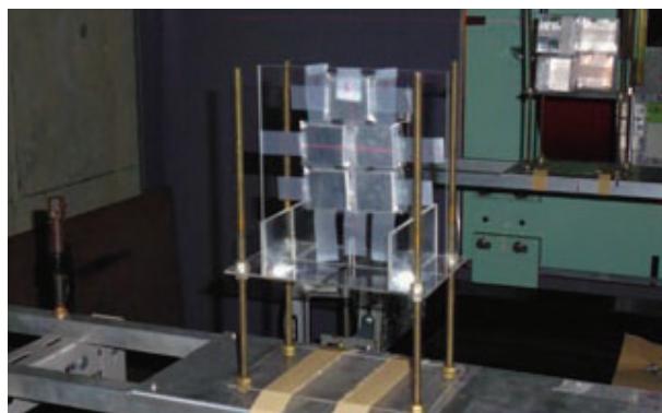
大阪大学核物理研究センターでの中性子放射化断面積測定の様子
