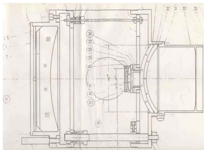
図 1 小林氏自筆による K1420 カメラ完成図面
