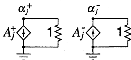
図7 \alpha_j^+ , \alpha_j^- の生成回路
