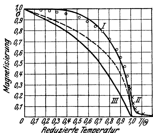
Fig. 4. Magnetisierung und Temperatur. I. Spontane Magnetisierung; Verfasser. — — Nach der Weiss'schen Theorie, O Beobachtung (P. Weiss und R. Forrer). II. Magnetisierung; H = 15000 Gauß. X Beobachtung (P. Weiss und R. Forrer). III. Magnetisierung; H = 10 Gauß ( 2n = 2 \cdot 10^6 , \theta = 634^\circ \text{K.} )
