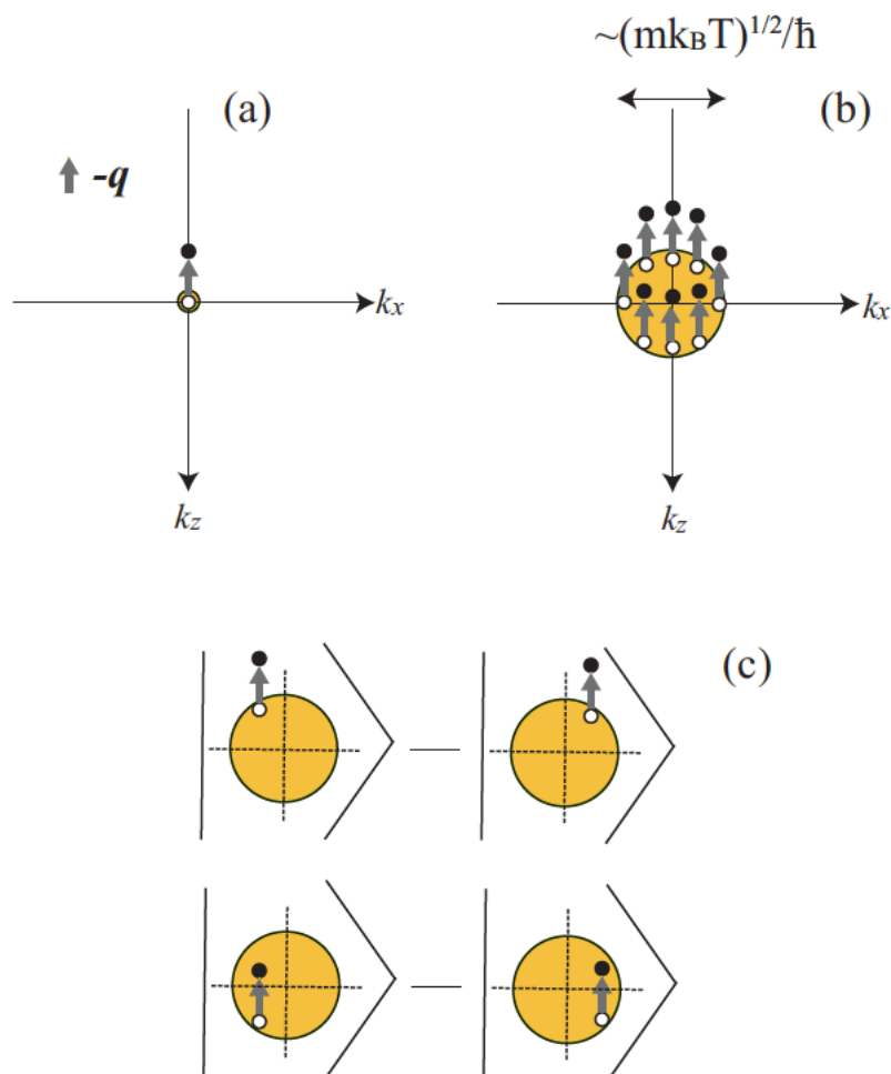
図 7: (a) T = 0 での自由ボース系の励起状態。白丸が \hat{a}_{\mathbf{k}+\mathbf{q}} に対応し、黒丸が \hat{a}_{\mathbf{k}}^\dagger に対応する。(b) 有限温度自由ボース系の励起状態。平衡状態では熱的ドブroy波長の逆数程度の波数までの状態が存在する。(c) 有限温度ボース系での横励起状態の例。温度が低ければ低いほど横励起状態の数は減少する。
