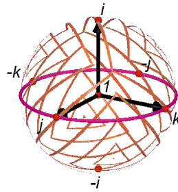
図 3: 単位四元数 1, i, j, k, -i, -j, -k の可視化
