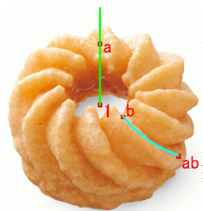
図 1: 四元数の積の直観的イメージ
