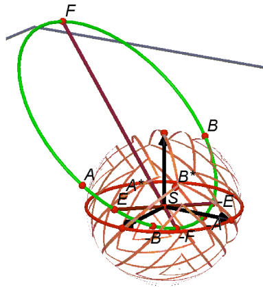
図2: S^3 の立体射影における大円 \overline{AB}
