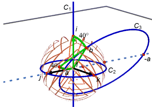
図 4: クリフォード平行
