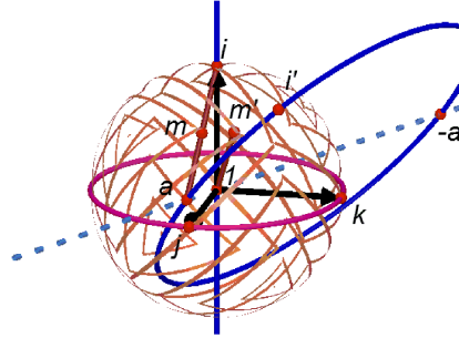
図 6: クリフォード平行の作図
