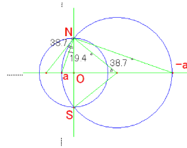
図 5: 中心角と円周角
