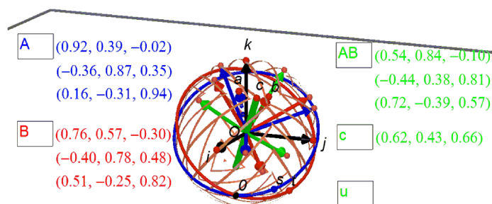
図 10: 軸の変化のスピン現象
