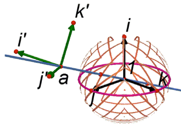
図 8: 単位四元数と SO(3) との関係
