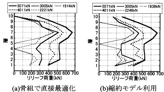
図 4 最適化 D によるリリーフ荷重分布
