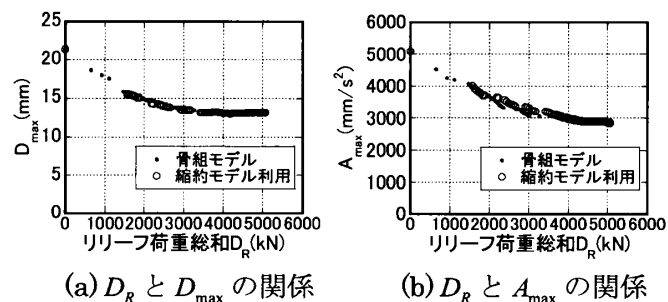
図 3 最適化 A による D_R と D_{\max} , A_{\max} の関係
