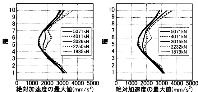
(a)骨組で直接最適化 (b)縮約モデル利用
