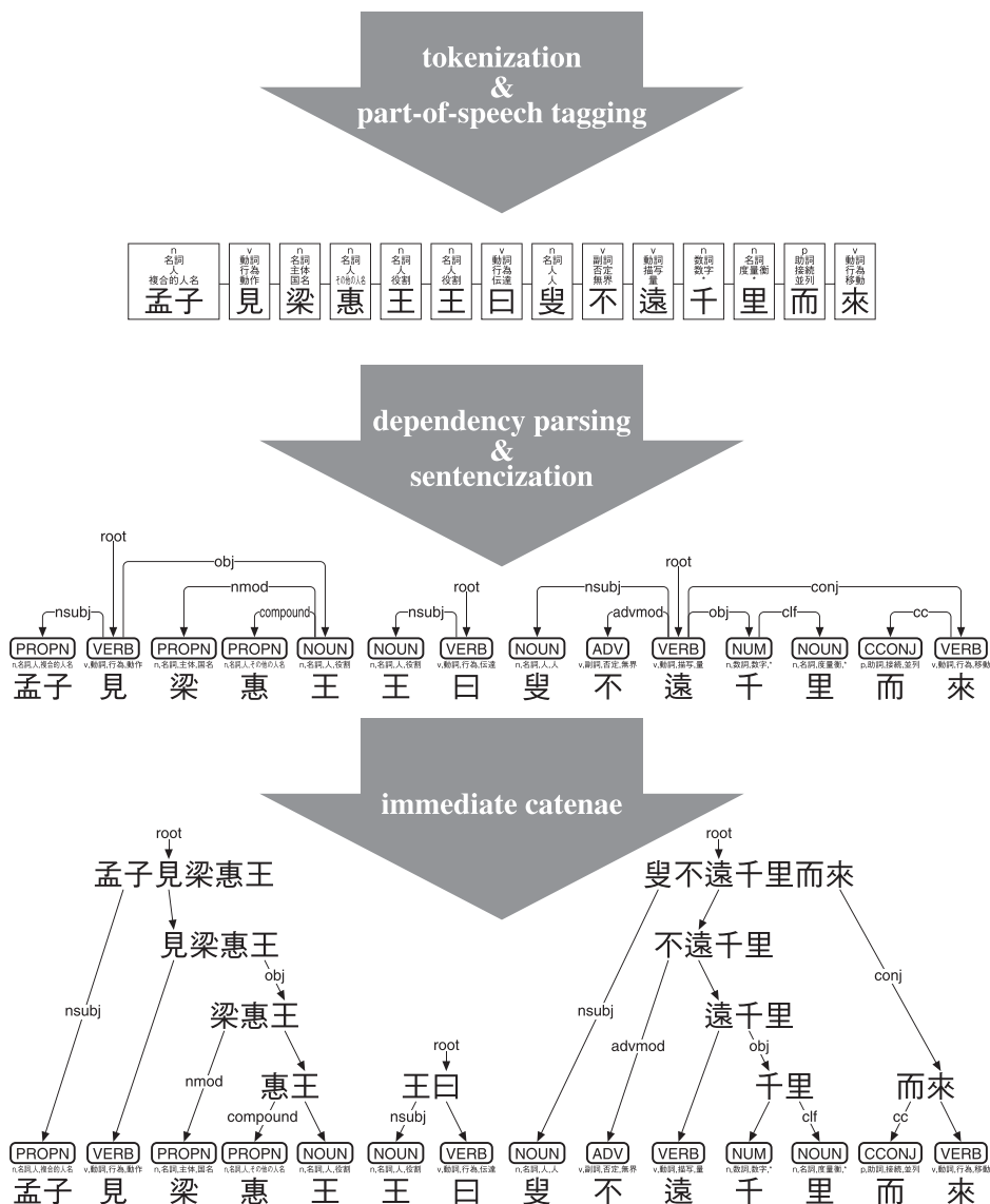
圖1 漢文の形態素解析・依存文法解析・直接構成鎖解析
