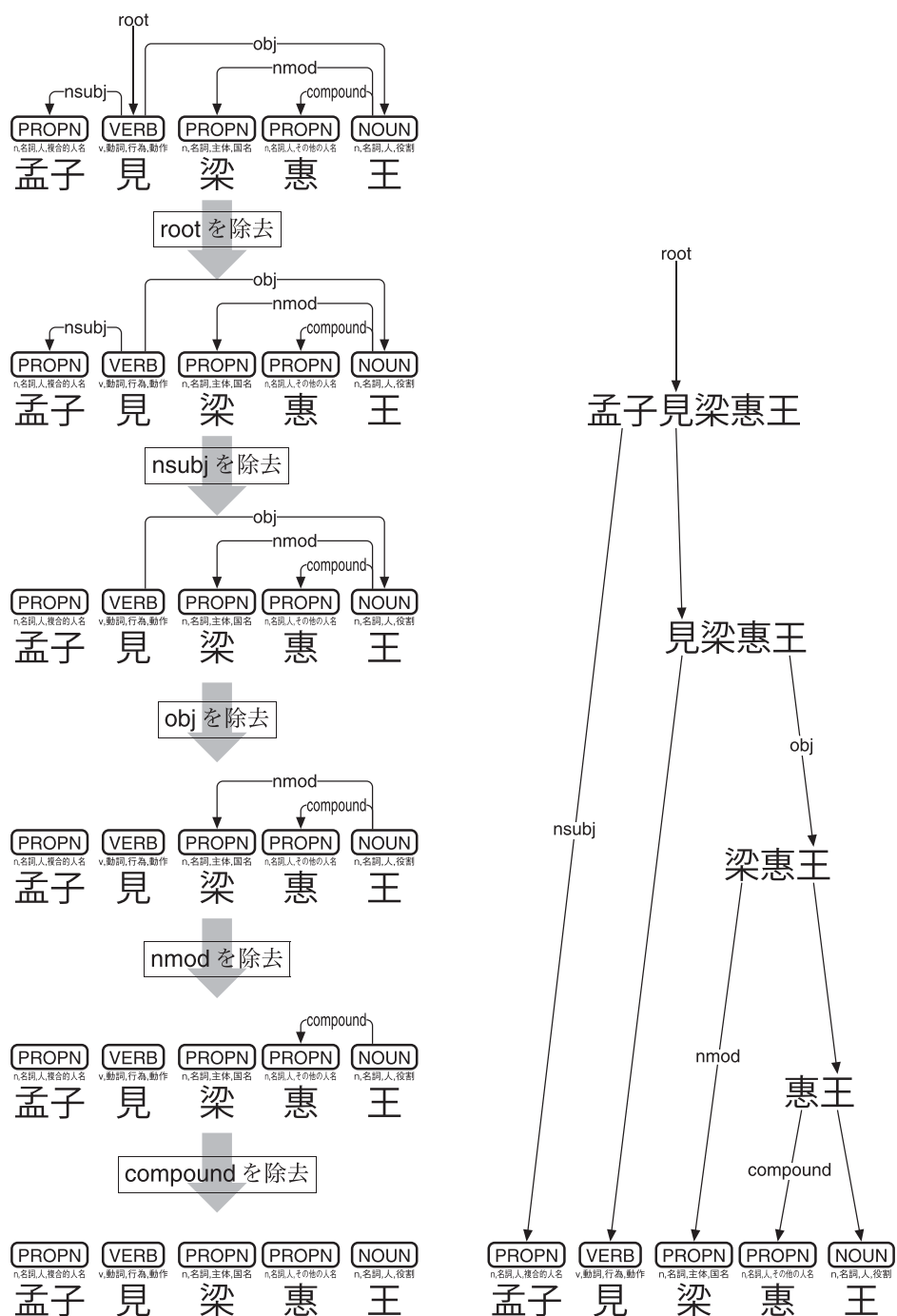
圖5 「孟子見梁惠王」の直接構成鎖解析
