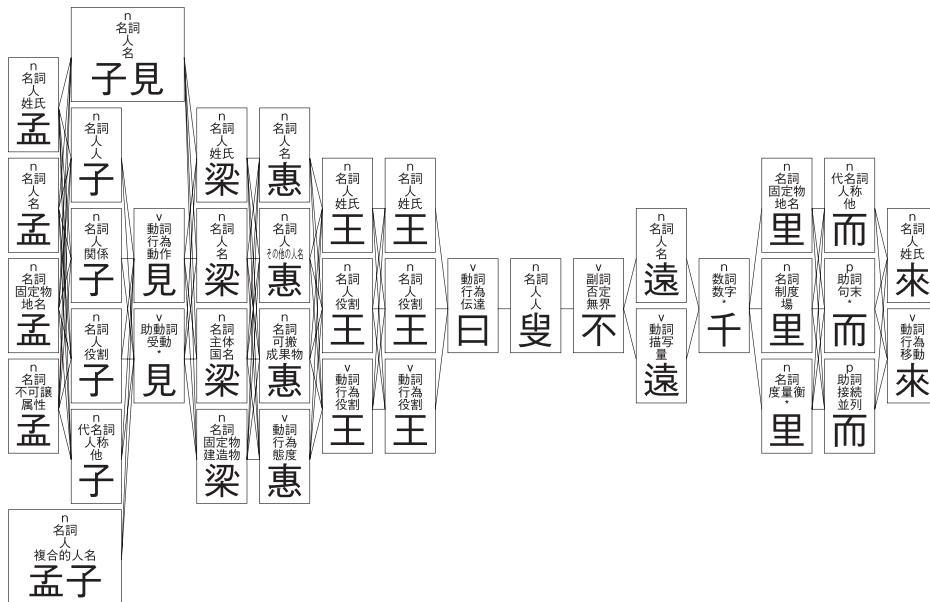
圖 2 CRF を用いた漢文の形態素解析
