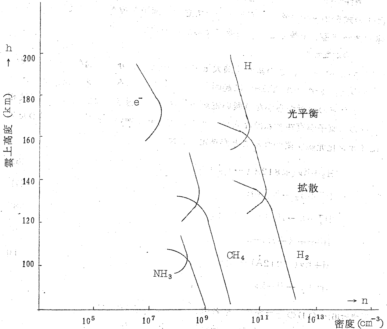
才 2 図 木星大気諸成分の解離と電離 ( H_2 以外は photochemical equilibrium を仮定)
