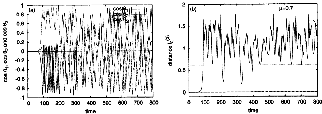
Figure 8: (a) 極渦の強さが \Gamma_1 = \Gamma_2 = 0.2\pi で赤道にある三点渦系 \cos \theta_1, \cos \theta_2, \cos \theta_3 の時間発展の様子. 初期摂動の方向は縮約系の方向に横断的な方向 \mu = 0.7 である. (b) 三点渦系環配置との距離を表す l_\zeta^{(3)} . 三点渦系環配置と極対称な三点渦系環配置に相当する l_\zeta^{(3)} = 0 と \frac{\sqrt{6}}{4} のところには点線を引いている.
