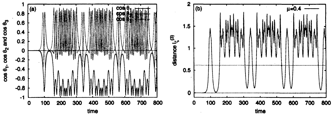
Figure 7: (a) 極渦の強さが \Gamma_1 = \Gamma_2 = 0.2\pi で赤道にある三点渦糸 \cos \theta_1 , \cos \theta_2 , \cos \theta_3 の時間発展の様子. 初期摂動の方向は縮約系の方に横断的な方向 \mu = 0.4 である. (b) 三点渦糸環配置との距離を表す l_\zeta^{(3)} . 三点渦糸環配置と極対称な三点渦糸環配置に相当する l_\zeta^{(3)} = 0 と \frac{\sqrt{6}}{4} のところには点線を引いている.
