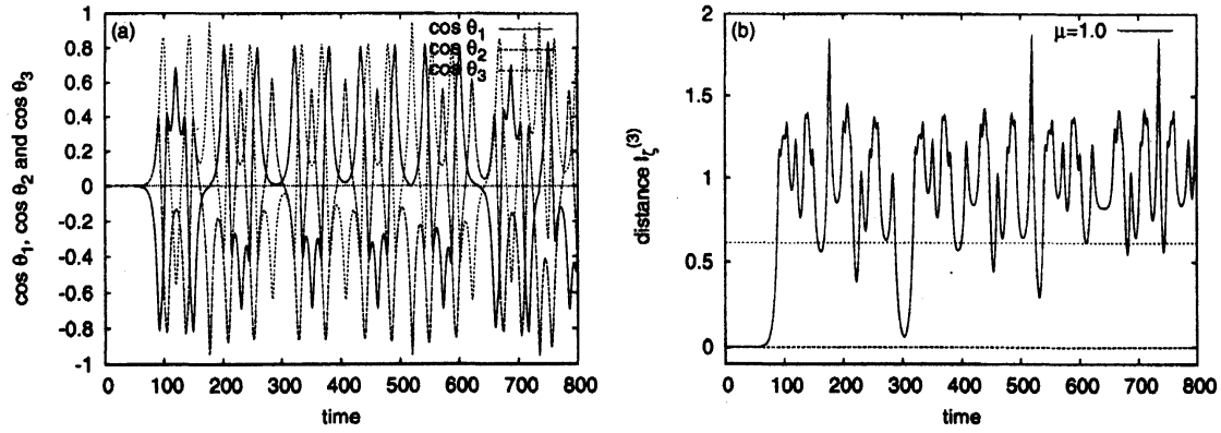
Figure 6: (a) 極渦の強さが \Gamma_1 = \Gamma_2 = 0.2\pi で赤道にある三点渦糸 \cos \theta_1 , \cos \theta_2 , \cos \theta_3 の時間発展の様子. 初期摂動の方向は縮約系の方に横断的な方向 \mu = 1.0 である. (b) 三点渦糸環配置との距離を表す l_\zeta^{(3)} . 三点渦糸環配置と極対称な三点渦糸環配置に相当する l_\zeta^{(3)} = 0 と \frac{\sqrt{6}}{4} のところには点線を引いている.
