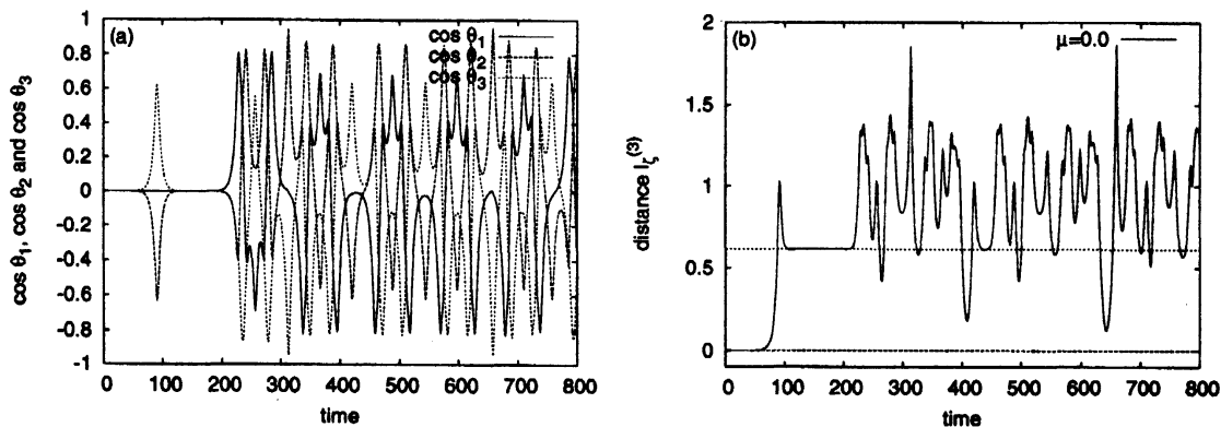
Figure 5: (a) 極渦の強さが \Gamma_1 = \Gamma_2 = 0.2\pi で赤道にある三点渦糸 \cos \theta_1 , \cos \theta_2 , \cos \theta_3 の時間発展の様子. 初期摂動の方向は \mu = 0.0 である. (b) 三点渦糸環配置との距離を表す l_\zeta^{(3)} . 三点渦糸環配置と極対称な三点渦糸環配置に相当する l_\zeta^{(3)} = 0 と \frac{\sqrt{6}}{4} のところには点線を引いている.
