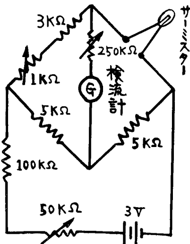
図6 ブリッジ回路
