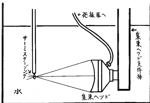
図8 サーミスターゾンデ法による集束ヘッド音 強度測定並びに特性検査
