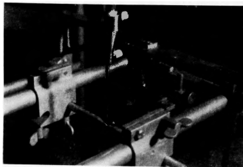
図4 第1号装置の集束ヘッド支持棒に3号ポインターを装着し機械的零点を測定
