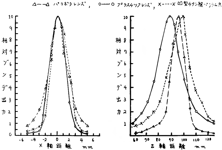
図9 サーマスターゾンデによる各種集束ヘッドの特性曲線
