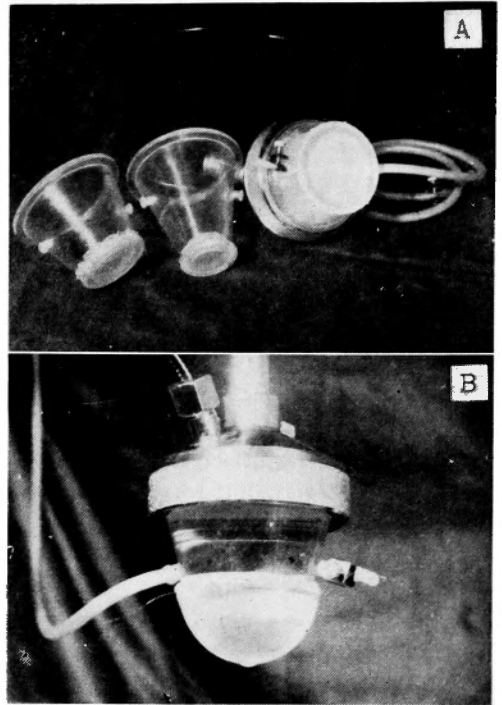
A : 集束ヘッドに装着深さ5 cm (右), 深さ8.5 cm (中), 深さ6 cm (左)。 B : 凹型チタン酸バリウム型集束ヘッドにカップ型照射槽を装着, 中に脱気水を満す。
