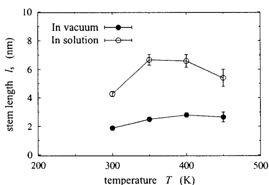
図 2: 真空中および溶液中における配向秩序構造のステム長の温度依存性。
