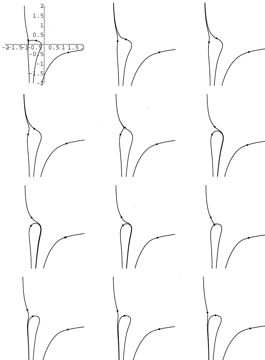
Figure A-4 : 変わり点 x = 0.471143 + 0.0498704 i の周り
