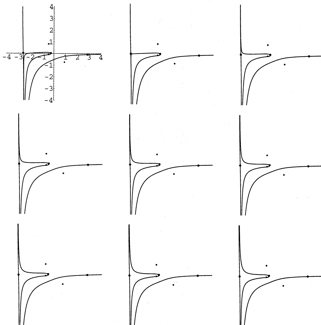
Figure A-7 : 直線 \operatorname{Re} x = 1.37 に沿って Stokes 曲線を横断
