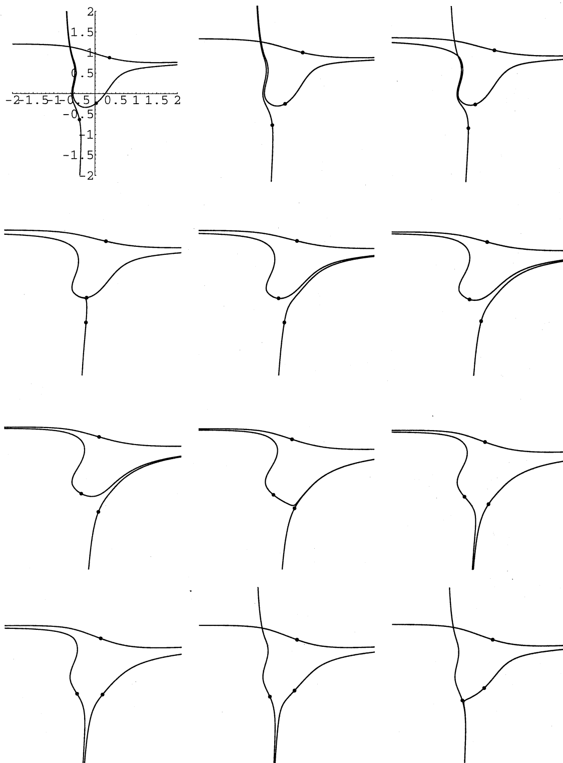
Figure A-3 : 変わり点 x = 0.32689 + 0.5109 i の周り
