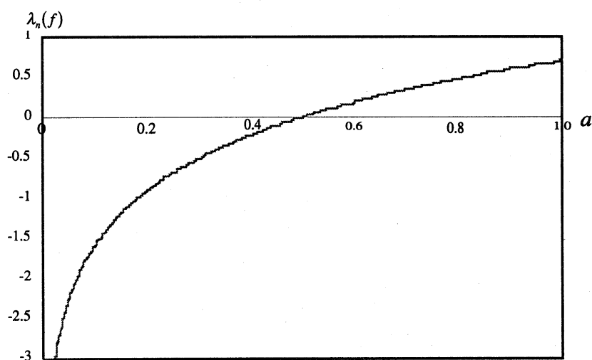
図4. パイこね変換のリアプノフ指数
