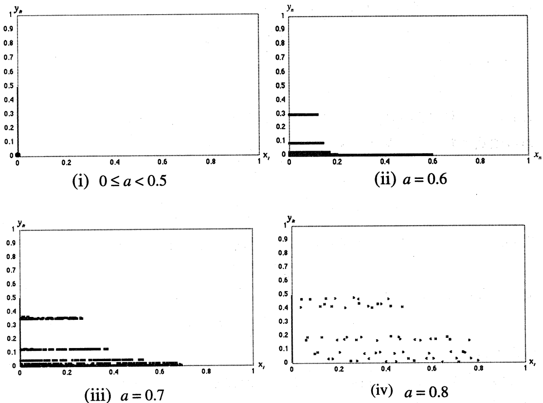
図1. パイこね変換の軌道図 (その1)
