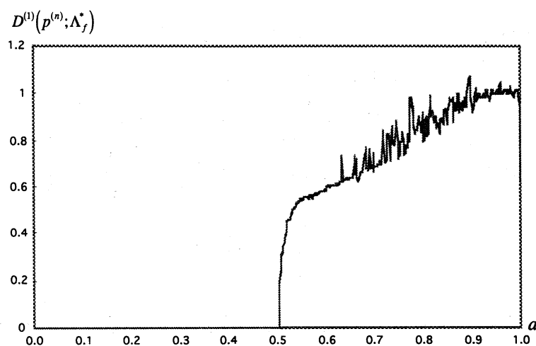
図3. パイこね変換のエントロピー型カオス尺度 D^{(1)}(p^{(n)}; \Lambda_f^*)
