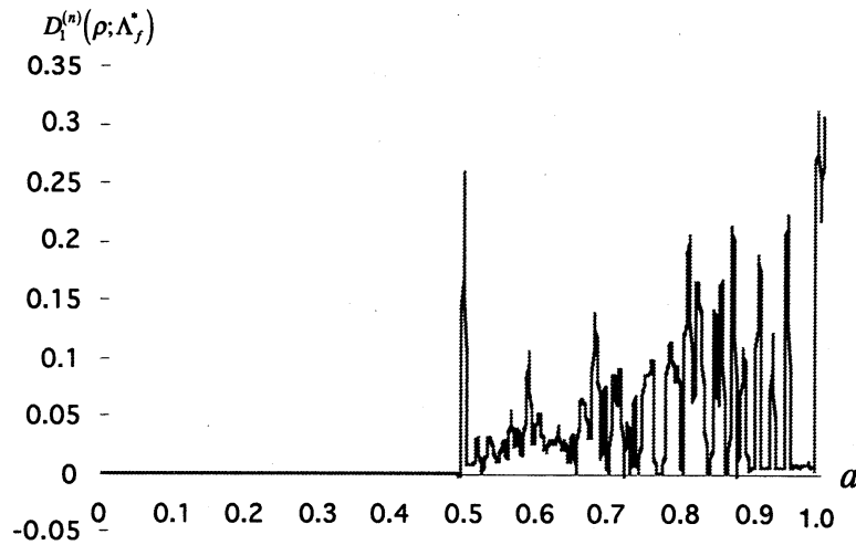
図5. パイこね型変換から導かれたスピン系の非線形チャンネル のカオス尺度 D_1^{(n)}(\rho; \Lambda_f^*) ( m=1000, n=2000 )
