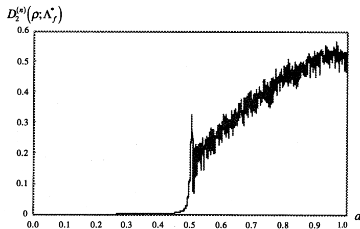
図6. パイこね型変換から導かれたスピン系の非線形チャンネル のカオス尺度 D_2^{(n)}(\rho; \Lambda_f^*) ( m=10, n=110 )
