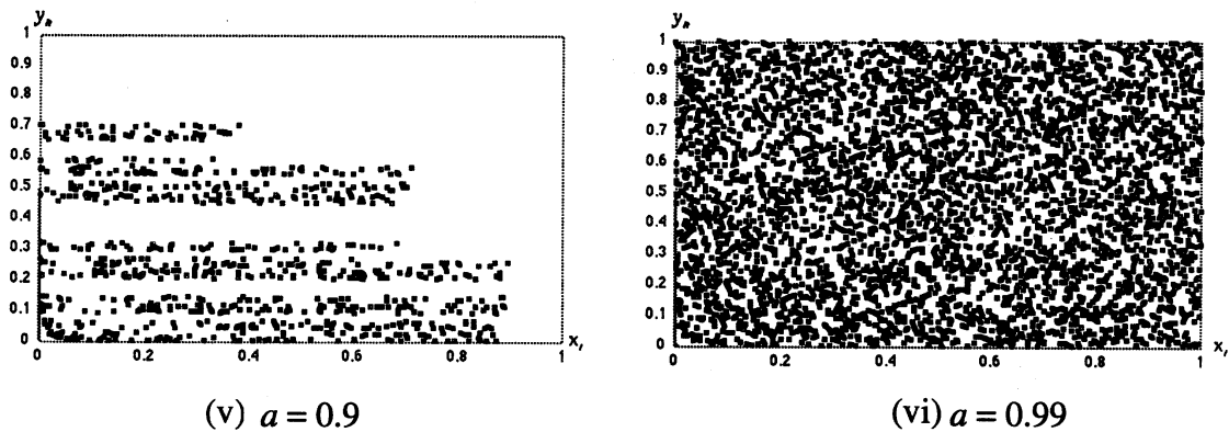
図2. パイコね変換の軌道図 (その2)
