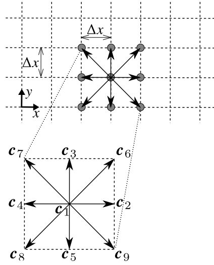
(a) D2Q9 model
