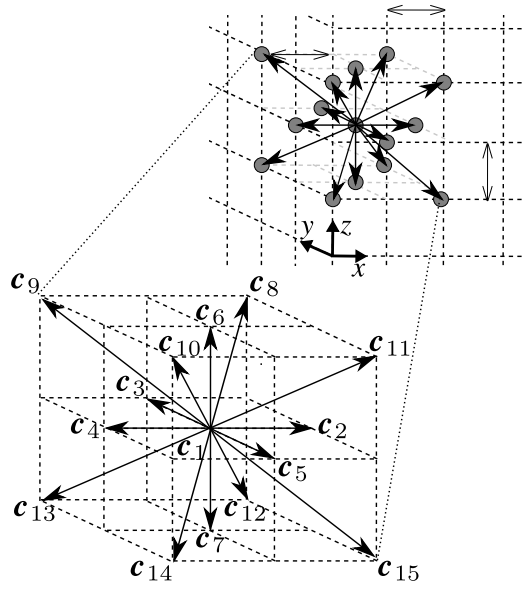
(b) D3Q15 model
